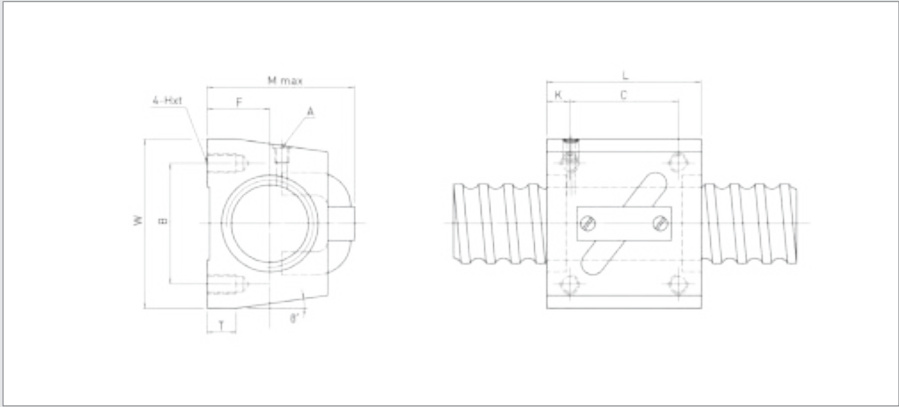
Block-Einzelmutter SSV für gerollte Kugelgewindespindeln
