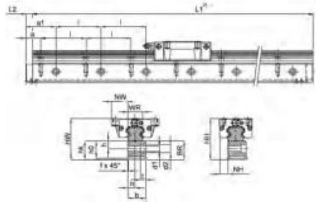
Laufwagen Modell HGW.. 2) Block type HGW.. 2)
